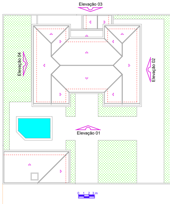
Implantação e Cobertura
